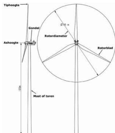
Afbeelding 3.1 Parameters windturbine
