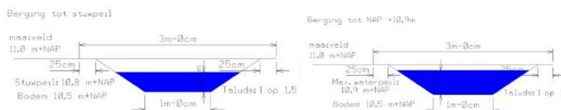
Figuur 13. Profiel wadi met waterpeil op stuwwiel NAP+10.80 m (links) en waterpeil op insteek NAP +10,9m (rechts)
